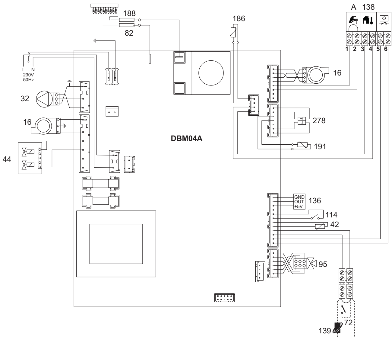
рис. 33 - Электрическая схема
